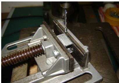
Werkstück ausspannen
