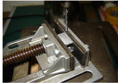
Werkstück einspannen
